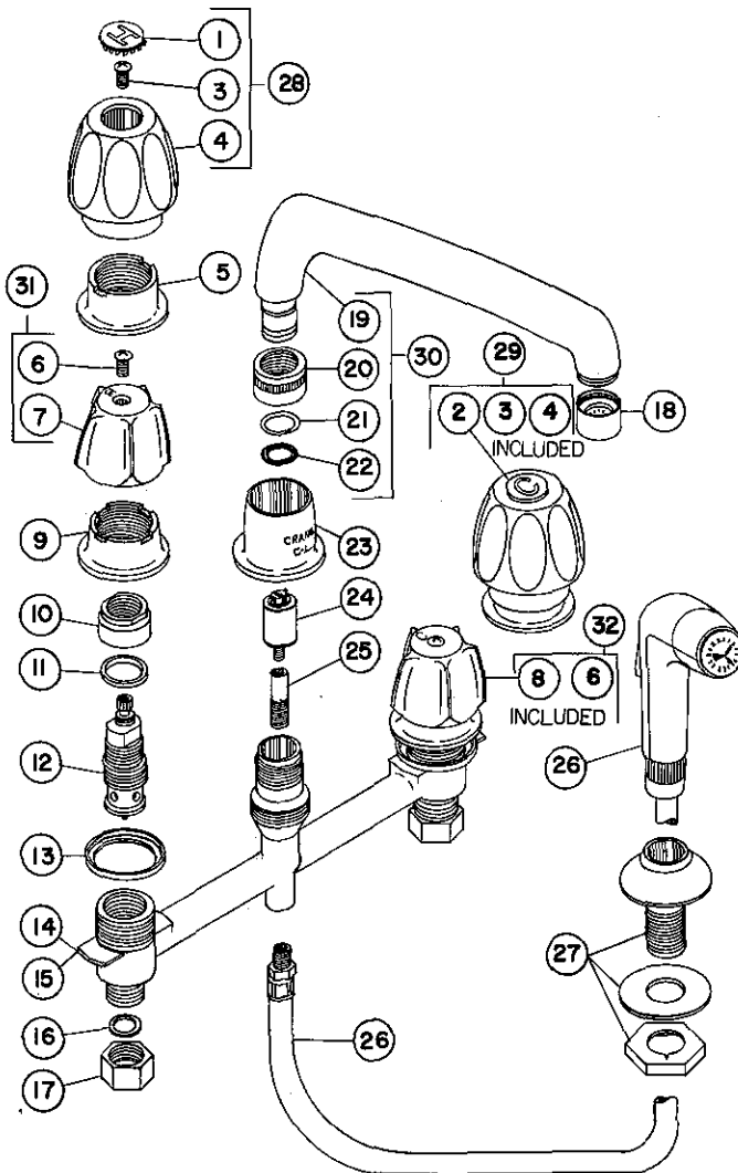
8-2720A 8-2724A ALL BRASS
