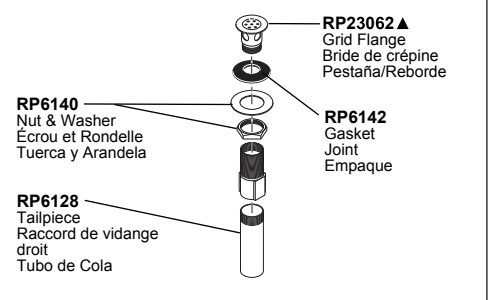
RP6346▲ Complete Grid Strainer Assembly Crépine complète Ensemble Complet del Colador con Rejilla
