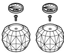
H41 Knob Handle Kit Manija Redonda Poignée Ronde
