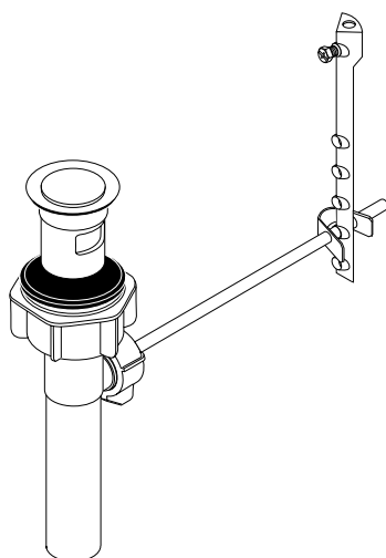
RP47416▲ Pop-Up Assembly Less Lift Rod Ensemble del Desagüe Automático Menos la Barra de Alzar Renvoi Mécanique Sans la Tige de Manoeuvre
