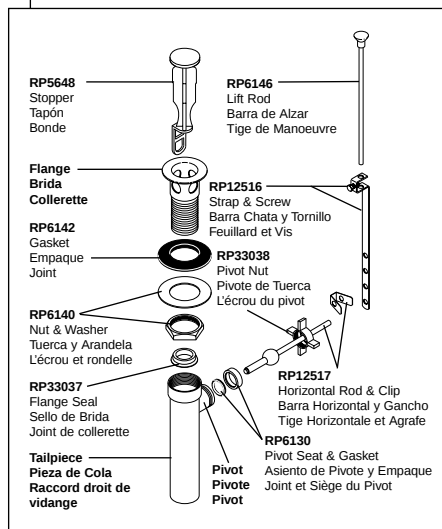
RP27575 Pop-Up Assembly Ensamble de Desagüe Automático Renvoi Mécanique
