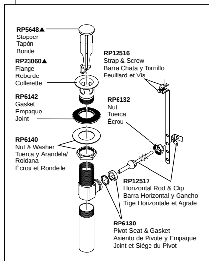
RP26533▲ Metal Pop-Up Assembly Ensamble de Metal del Desagüe Automático Renvoi Mécanique en Métal
