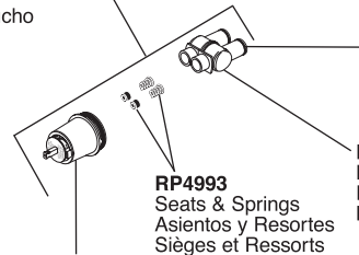
RP46070 Cap Assembly Ensamble de Tapón Soupape
