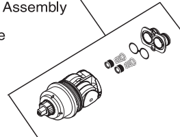
RP12630▲ For Longer Screws Para Tornillos Más Grandes Pour Vis Plus Longues
