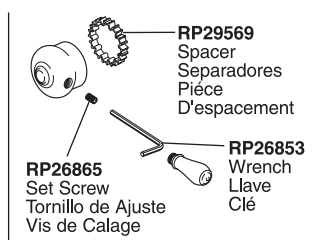
H778▲ Handle Kit Juego de herrajes de la Manija Manette en kit
