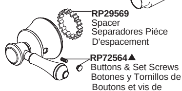
H797▲ Handle Kit Juego de herrajes de la Manija Manette en kit
