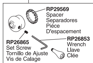
H778▲ Handle Kit Juego de herrajes de la Manija Manette en kit
